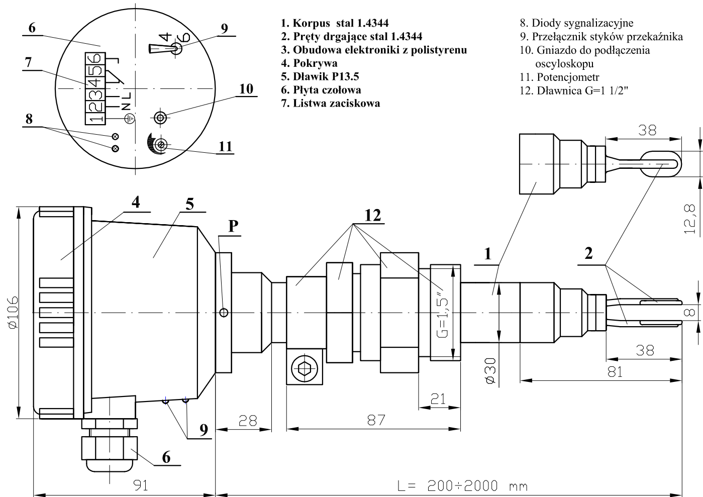
Rys. 1. Wibracyjny sygnalizator poziomu WSP-34D
