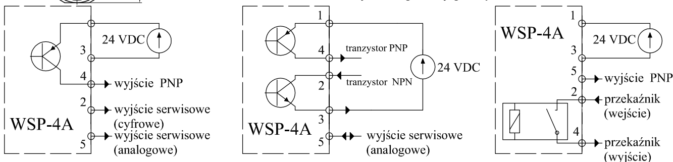
Rys. 2. Sposoby podłączenia
