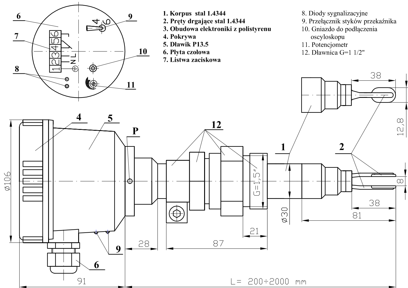
Rys. 1. Wibracyjny sygnalizator poziomu WSP-4D
