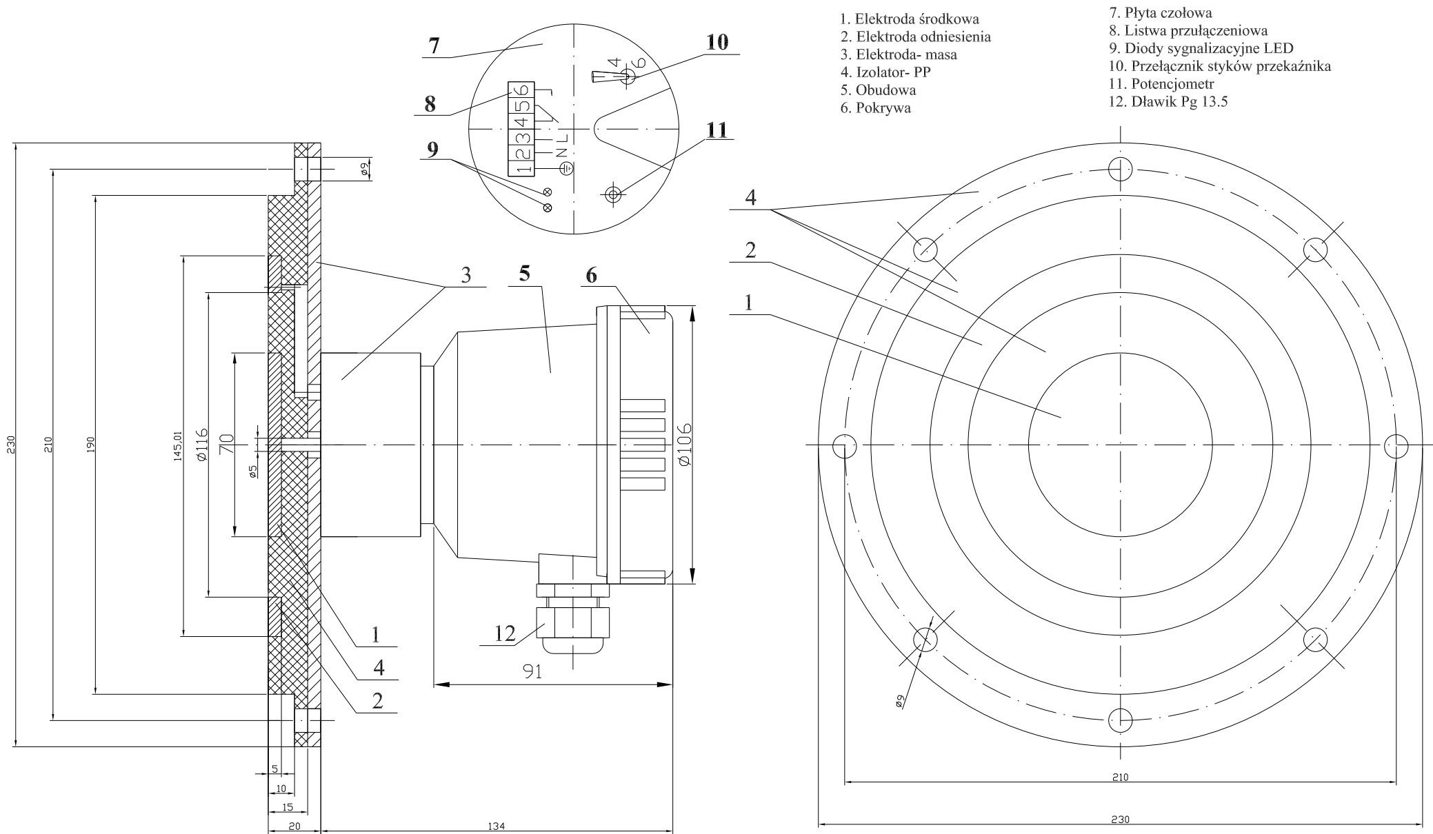
Rys. 1. Pojemnościowy sygnalizator poziomu CSP-7
