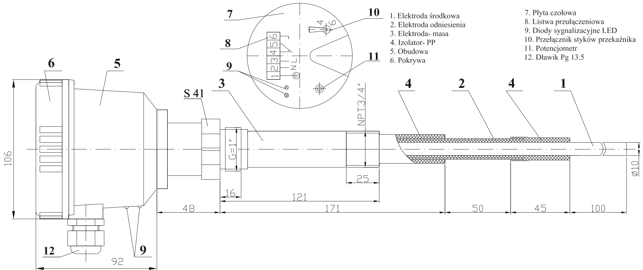
Rys. 1. Pojemnościowy sygnalizator poziomu CSP-8 do materiałów sypkich.
