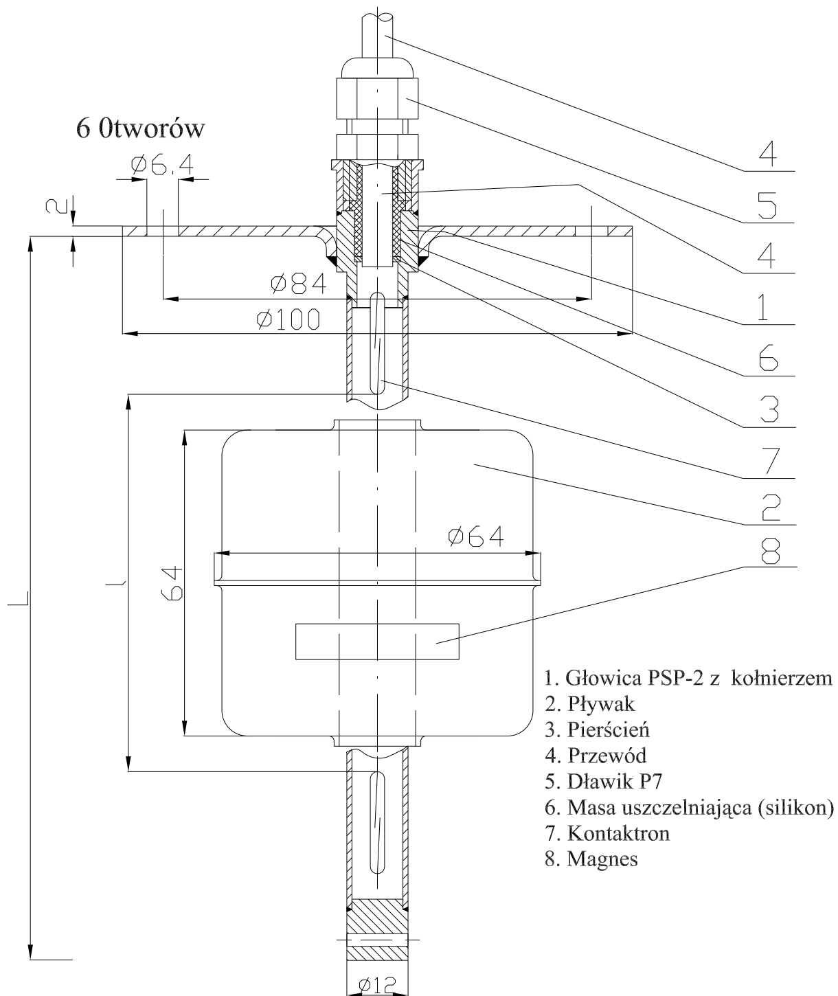
Pływakowy Sygnalizator Poziomy PSP-2.2-1-W4-K-24-D-
