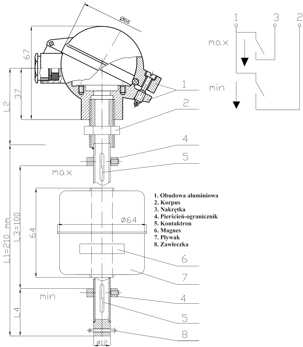
Pływakowy Sygnalizator Poziomu PSP-2.2-1-W4-G-24-O-
