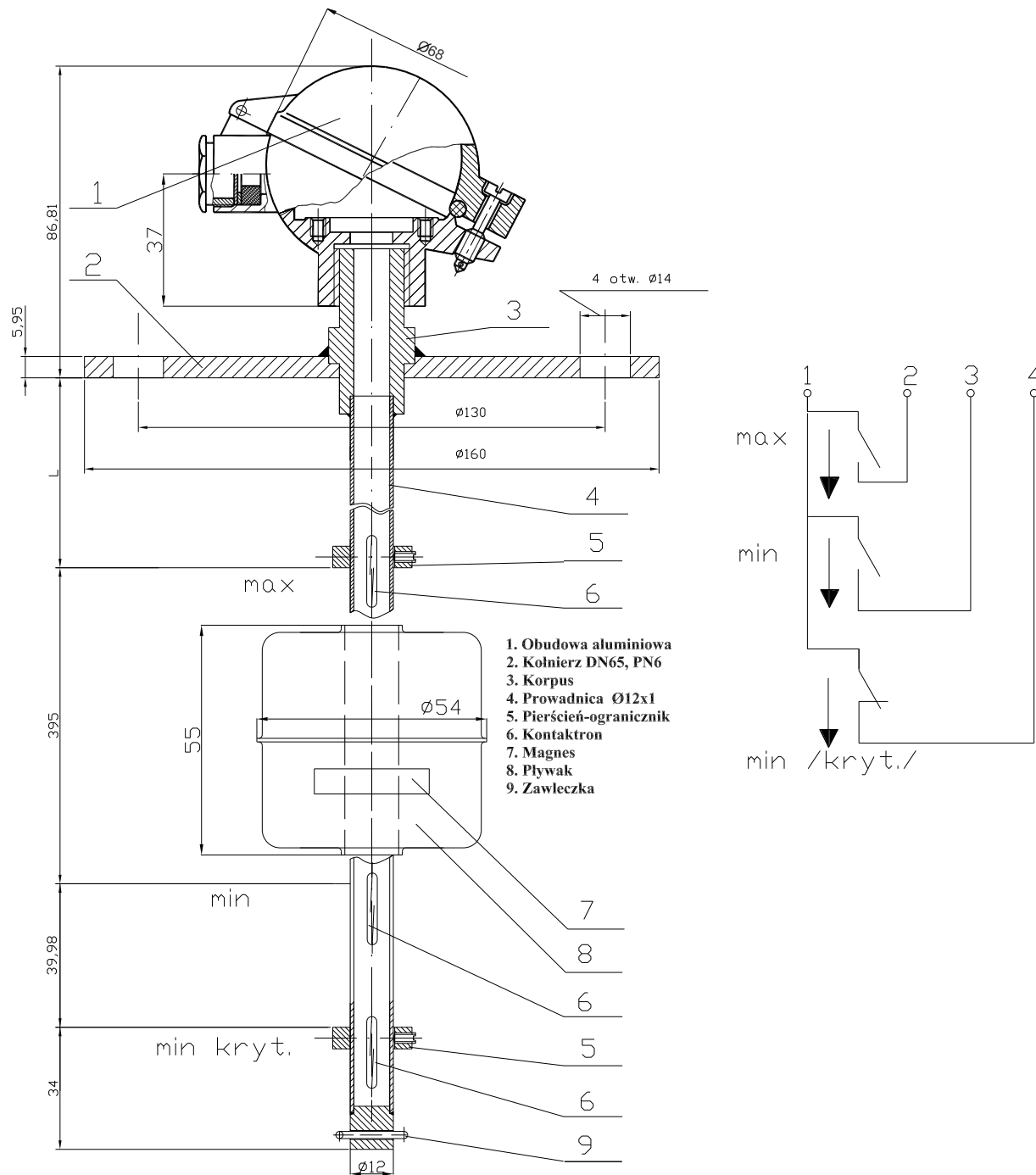
Pływakowy sygnalizator poziomu PSP-2.2-1-W3-K-24-O-(3kontaktrony)
