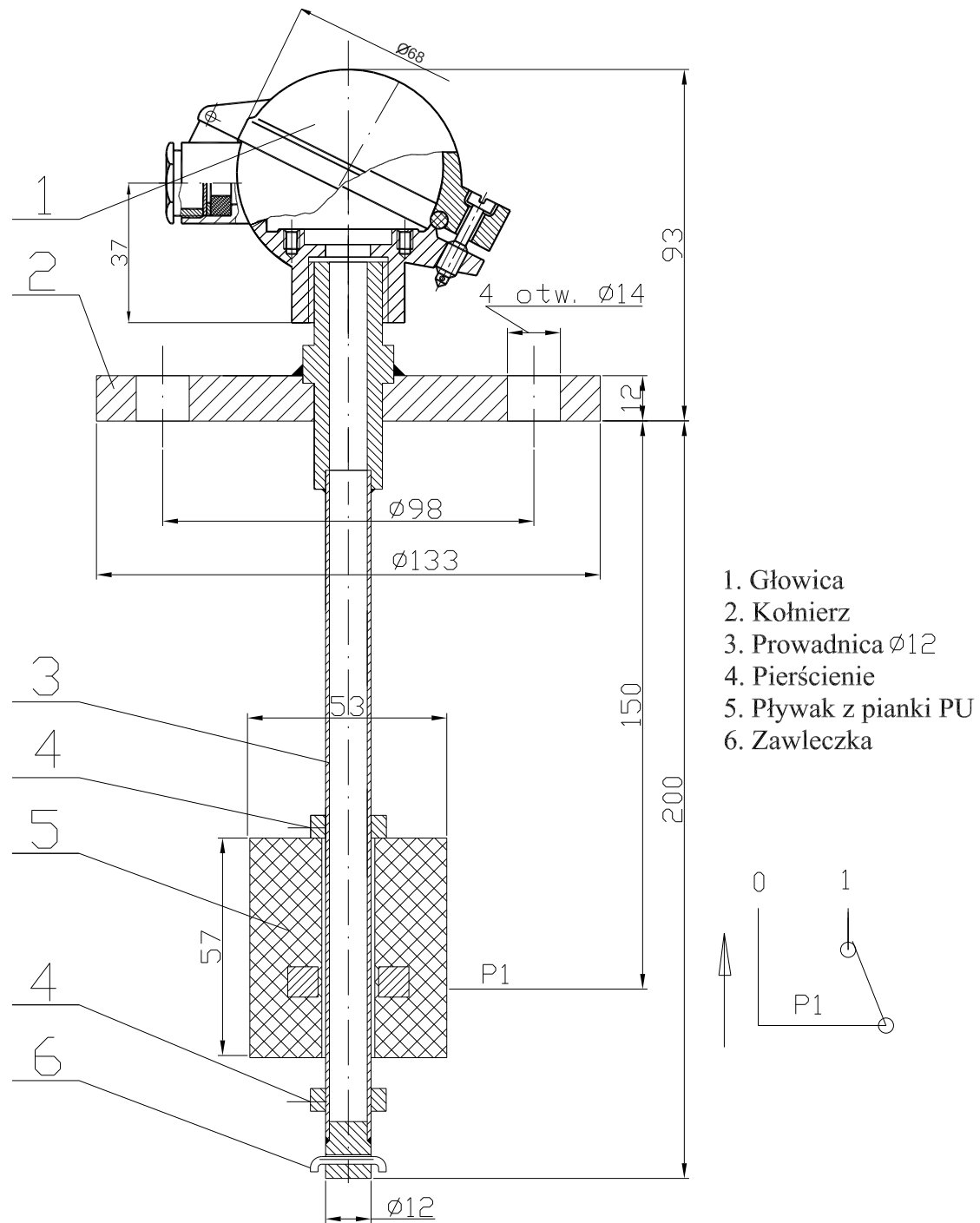
Pływakowy sygnalizator poziomy PSP-2.2-1-W3-K-24-O-(1kontaktron)
