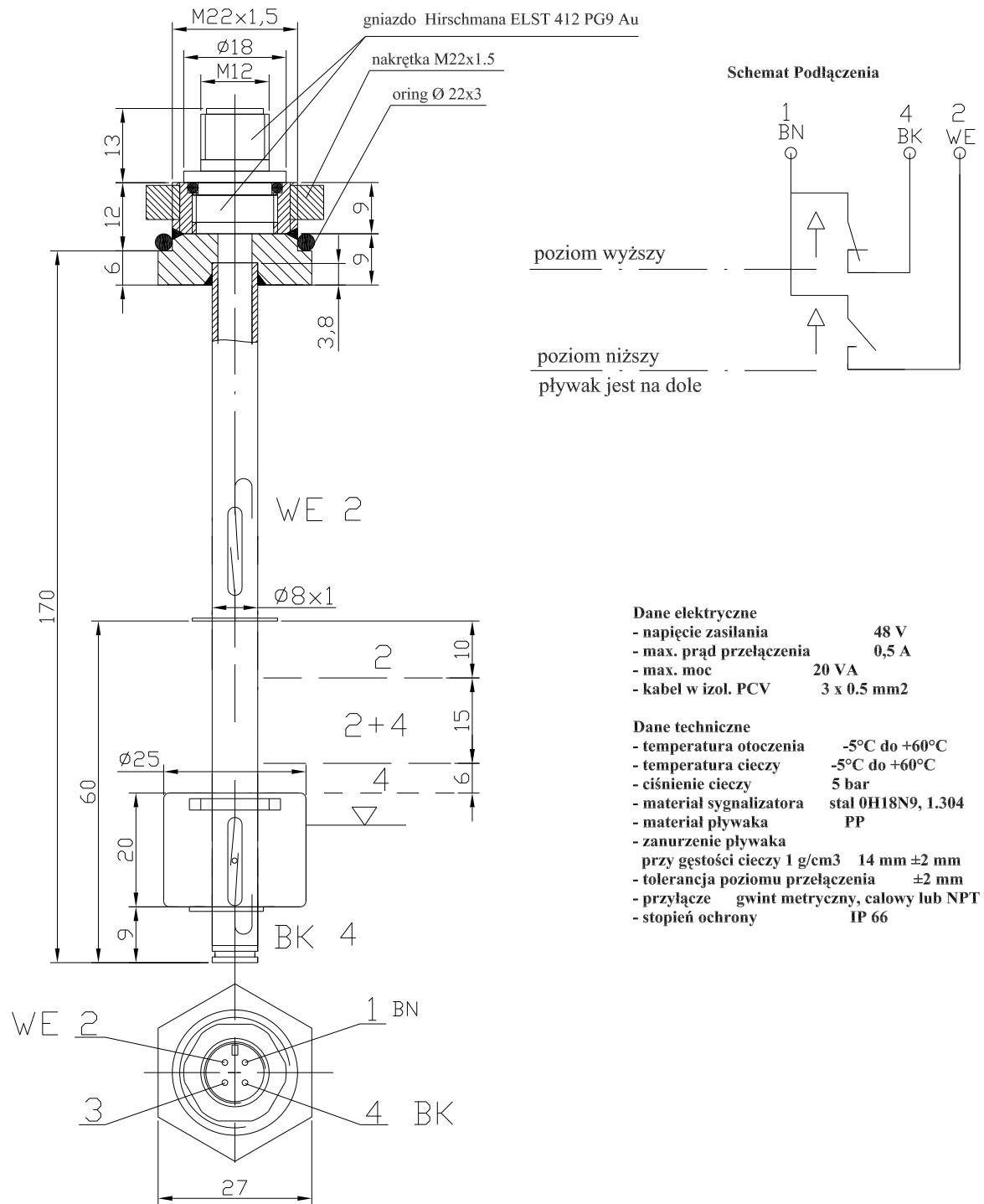
Pływakowy sygnalizator poziomy PSP-2.1-1-W1-G-48-G-
