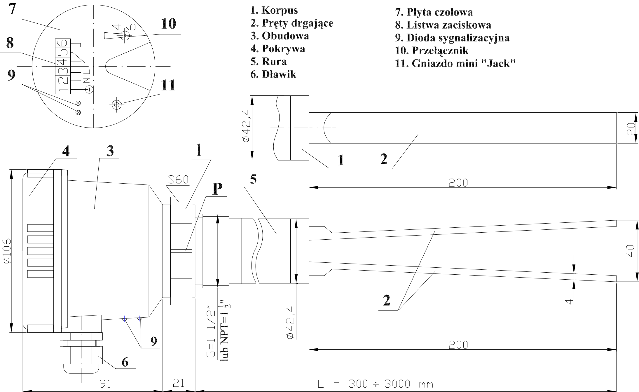
Rys. 1. Wibracyjny sygnalizator poziomu WSP-1B
