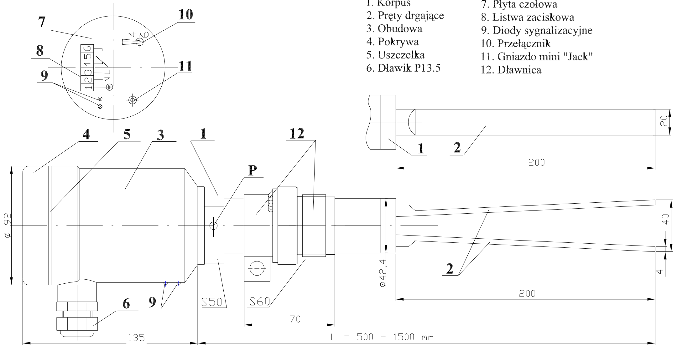
Rys. 1. Wibracyjny sygnalizator poziomy WSP-1D
