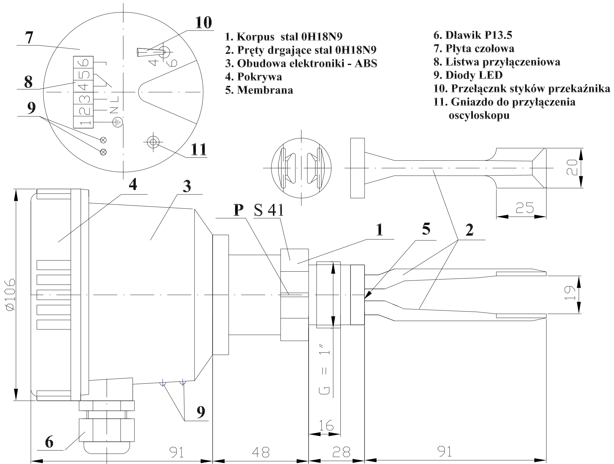
Rys. 1. Wibracyjny sygnalizator poziomy WSP-2A
