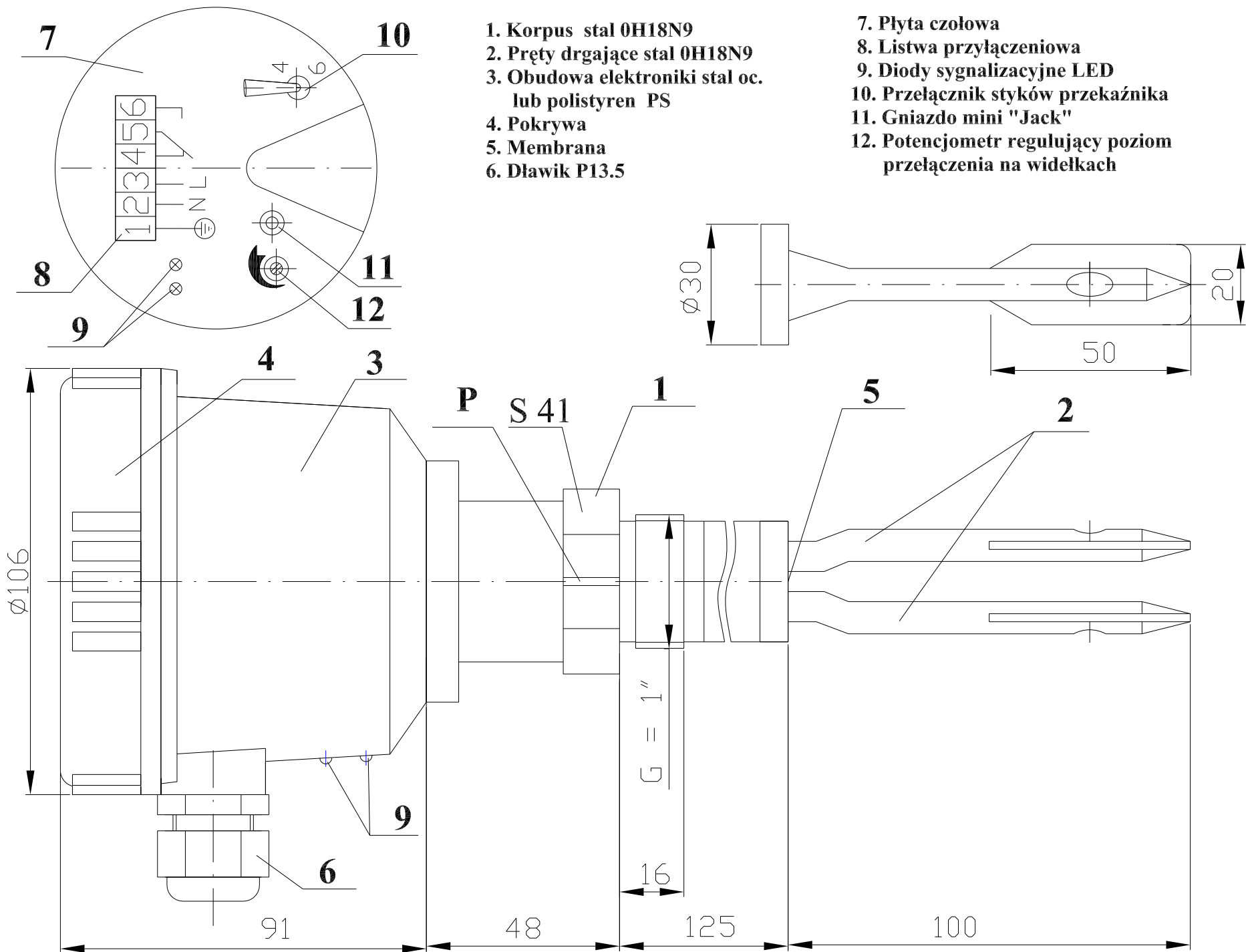
Rys.1. Wibracyjny sygnalizator poziomy WSP-3A
