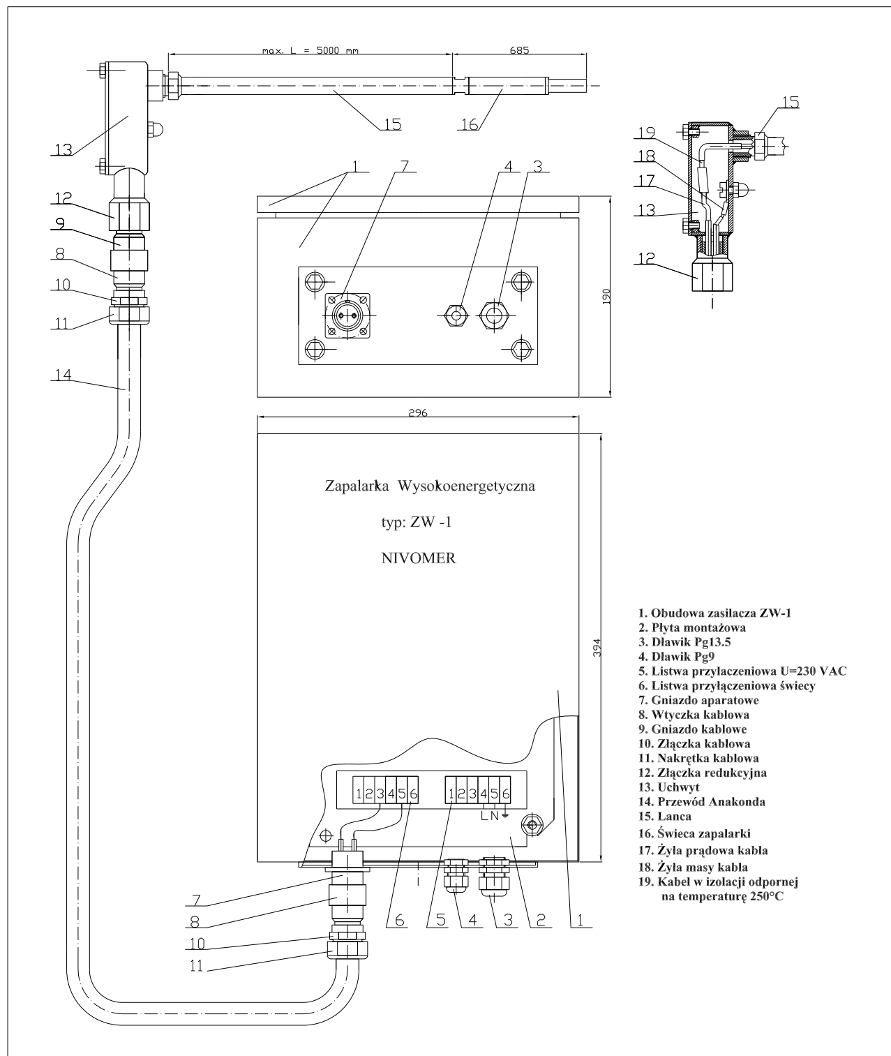
Rys. 1. Zapalarka wysokoenergetyczna ZW-1
