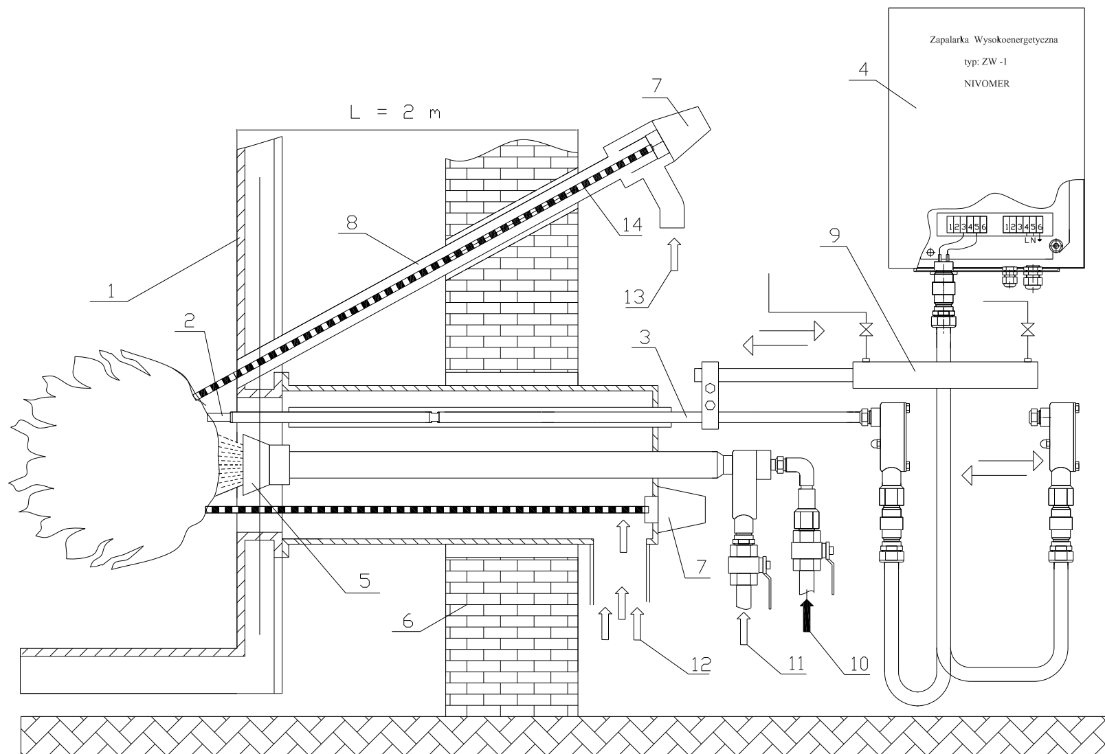
Rys. 5. Układ rozpalkowy kotła fluidalnego
